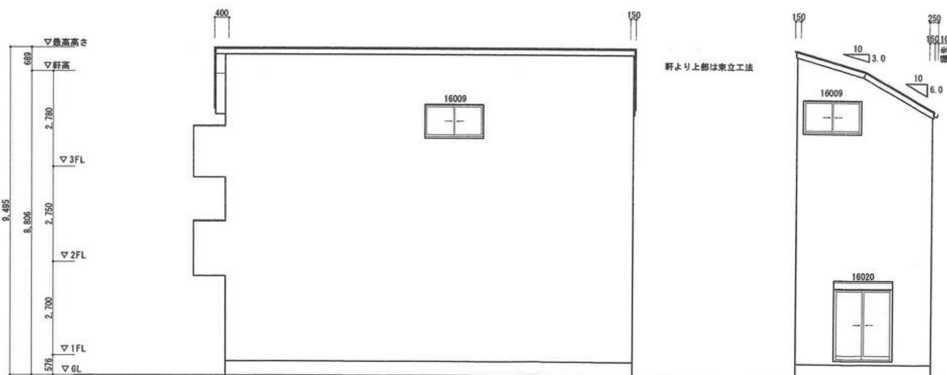
南立面図
