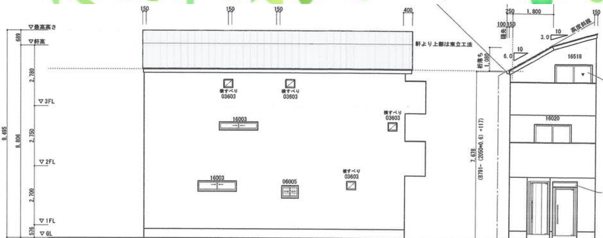
北立面図
