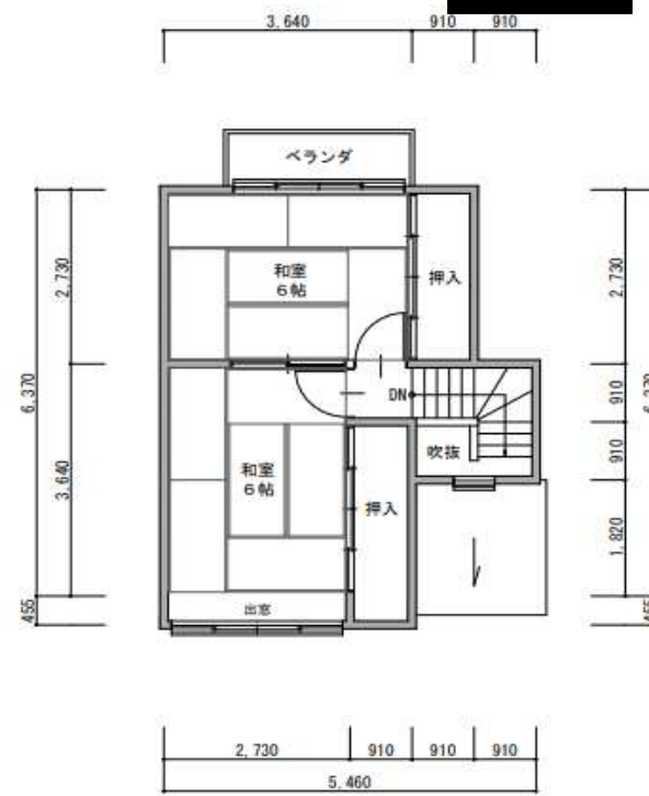
2階平面図
